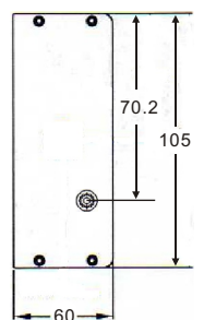
側視圖 (2.3英吋)
