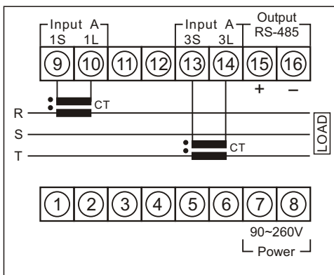
3P3W (PW-3A)
