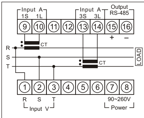
3P3W (PW-3VA)
