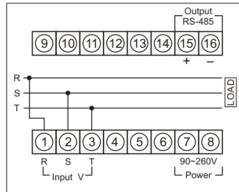
3P3W (PW-3V)
