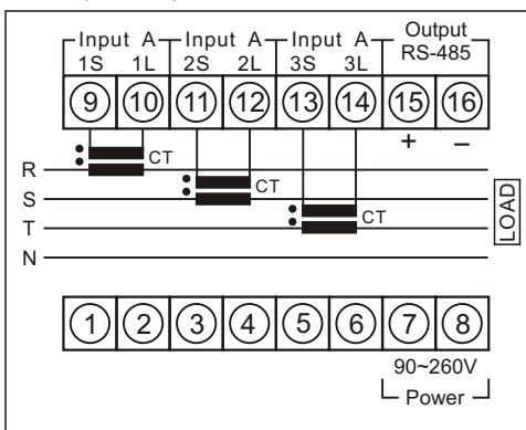
3P4W (PW-3A)
