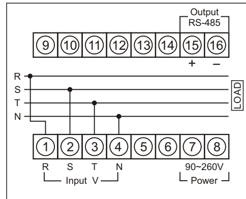
3P4W (PW-3V)
