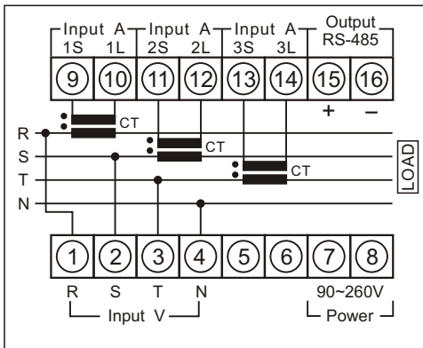
3P4W (PW-3VA)
